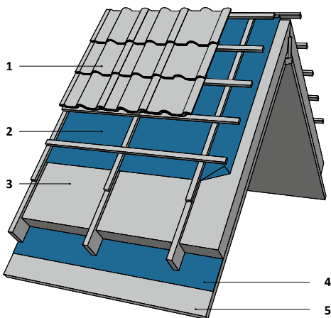
Obr. 1. Uložení vrstev v případě standardně oteplené šikmé střechy s užitkovým podkrovím: 1. vlastní střešní krytina, 2. pojistná hydroizolační vrstva – paropřepustná fólie STROTEX, 3. tepelně izolační vrstva 4. Paroizolace – paroizolační fólie STROTEX, BUDFOL nebo EKOFOL, 5. desky k-g.
