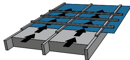
Obr. 4. Odvětrání prostřednictvím jedné odvětrací spáry – postačující v případě použití vysoce propustných membrán (2).
